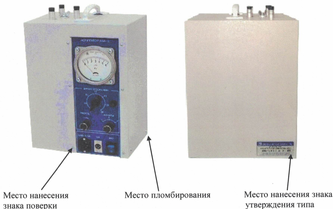
Рисунок 1 – Общий вид аспиратора АВА 3
